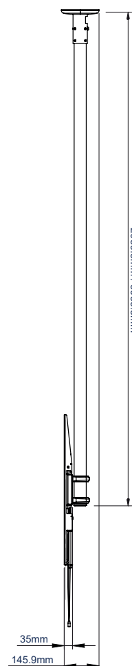
VUE DE CÔTÉ BT8448-200
